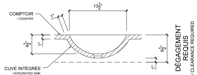
VUE EN COUPE / SECTION VIEW
