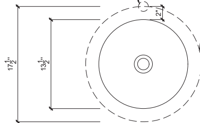
VUE EN PLAN / PLAN VIEW
