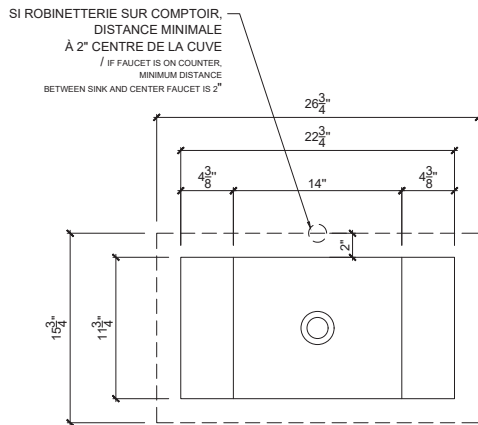
VUE EN PLAN / PLAN VIEW
