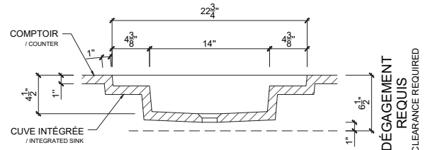
VUE EN COUPE (DE FACE) / SECTION VIEW (FACE)
