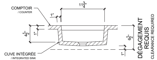
VUE EN COUPE (DE CÔTÉ) / SECTION VIEW (SIDE)
