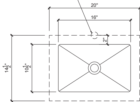
VUE EN PLAN / PLAN VIEW
